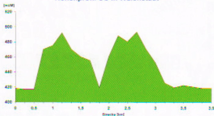
Höhenprofil CC in Walenstadt
